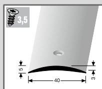
501 M Übergangprofil 40 mm Aluminium mittig versenkt gebohrt inkl. Dübel + Schrauben
