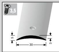
500 M Übergangprofil 30 mm Aluminium mittig versenkt gebohrt inkl. Dübel + Schrauben
